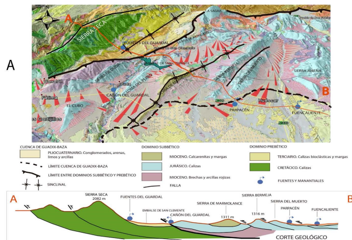
FIGURA 3.- A) MAPA GEOLÓGICO DE HUÉSCAR Y SAN CLEMENTE; DISTRIBUCIÓN DE LAS SIERRAS PREBÉTICAS Y SUBBÉTICAS. DELIMITACIÓN DE LA CUENCA DE GUADIX-BAZA (GEOPARQUE) B) SUPERPOSICIÓN EN ESCAMAS DE ESTOS DOS DOMINIOS. SITUACIÓN DE LOS PRINCIPALES MANANTIALES DE LA REGIÓN.
